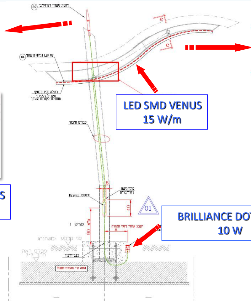
חתך 1-1 - עמוד K1
